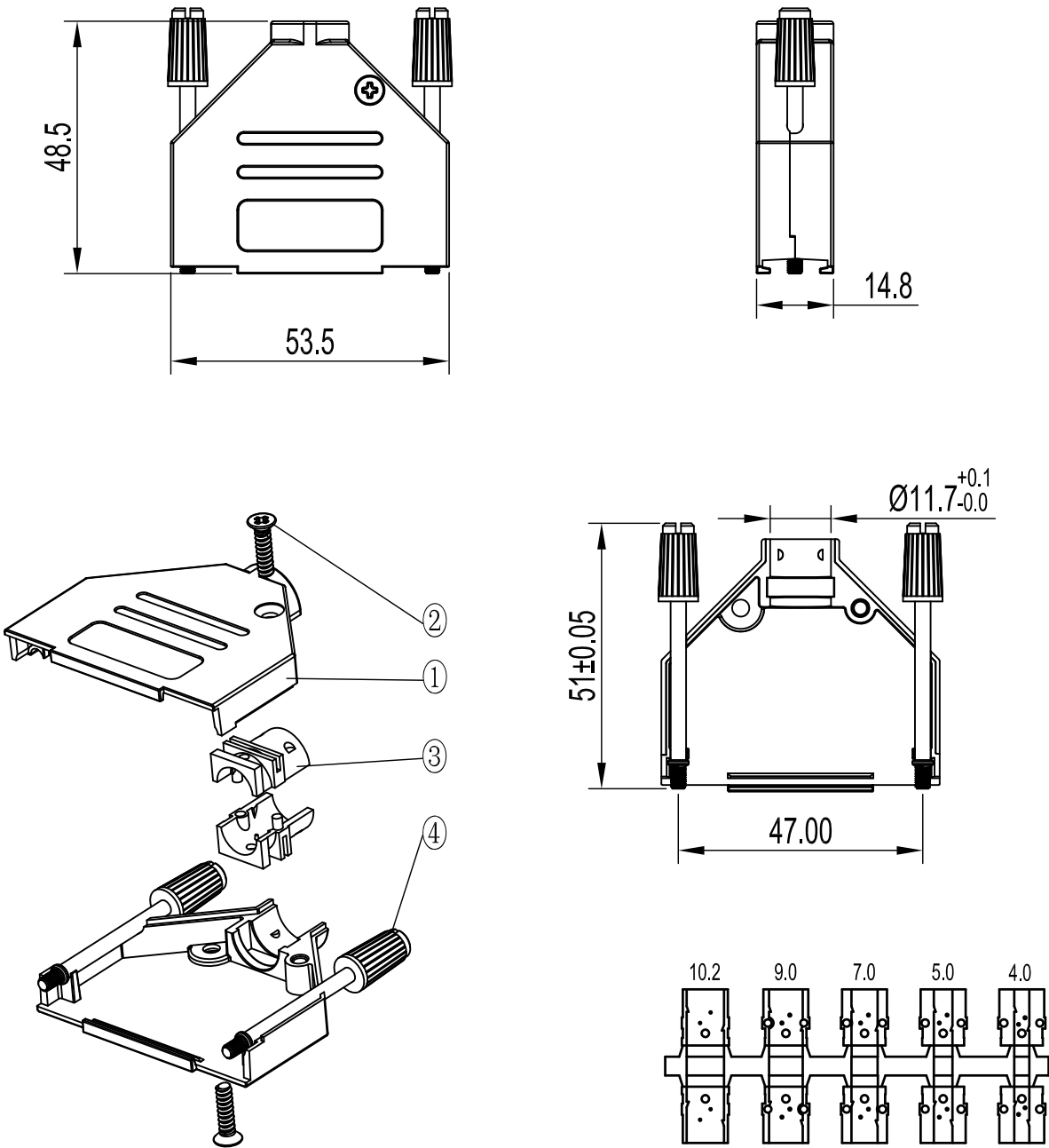
Grommet Set
